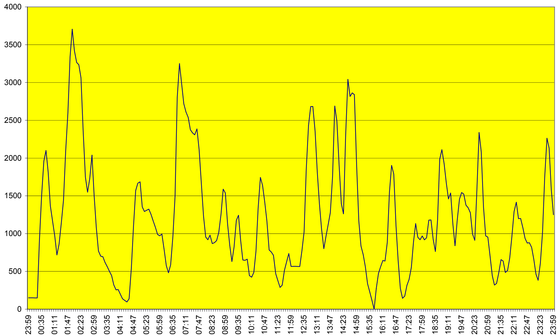
Pomiar TOC w surowych ściekach browarniczych w ciągu 1 doby
